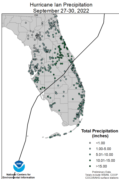
Ilustrasyon 9. Lapli Siklòn Ian (an pous) nan Eta Florid Sous: Sant Nasyonal pou Enfòmasyon Anviwònmanal, https://www.ncei.noaa.gov/access/monitoring/monthly-report/national/202209/supplemental/page-5
