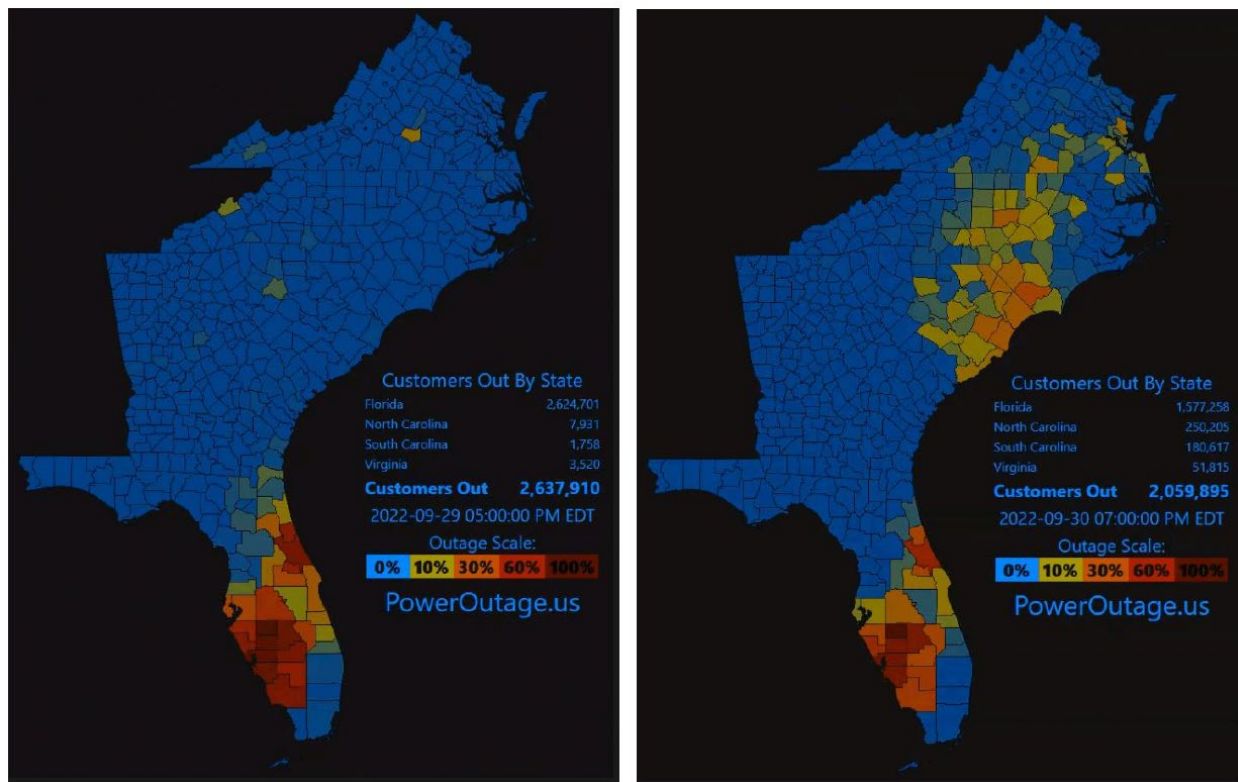
Ilistrasyon 6. Kat Geyografik pou Pann Kouran nan dat 29 septanm 2022 (agoch) ak 30 septanm 2022 (adwat)
