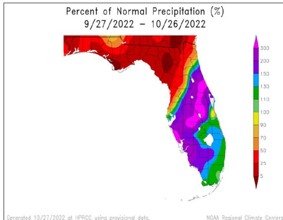
Ilistrasyon 3. Pousantaj Lapli Nòmal ki te Obsève soti nan dat 27 septanm pou rive 26 oktòb 2022 Sous: Sant Klima Rejyonal NOAA ke Sant pou Klima Florid nan Inivèsite Eta Florid la te adopte apati de Rapò sou Siklòn lan, https://climatecenter.fsu.edu/images/docs/Hurricane_lan_Report.pdf
