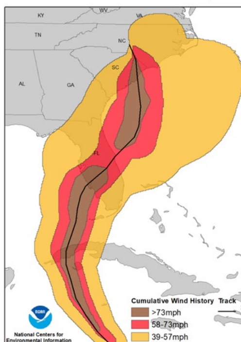
Illistrasyon 2. Istwa Van ak Wout Siklòn Ian Sous: Sant Nasyonal pou Enfòmasyon Anviwònmantal, https://www.ncei.noaa.gov .
